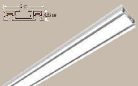
CT-9810 1 Metre ULTRA İNCE 0,55 cm CT-9811 2 Metre ULTRA İNCE 0,55 cm CT-9812 3 Metre ULTRA İNCE 0,55 cm
